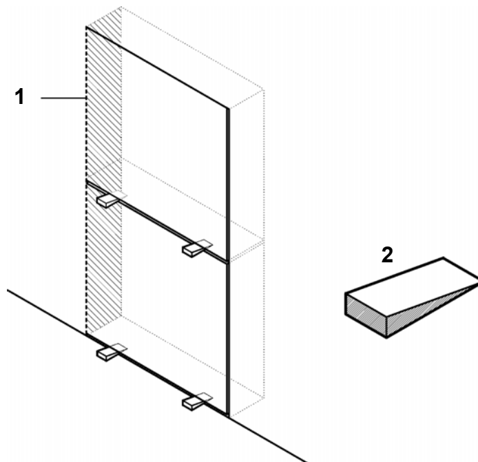
Рис. 6-16 Использование клиньев
