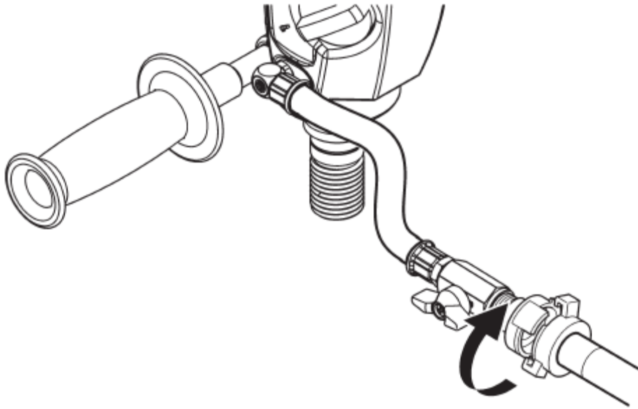
Подключение к линии подачи воды
