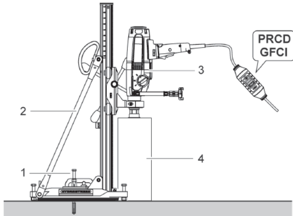
Малогабаритная установка колонкового бурения
