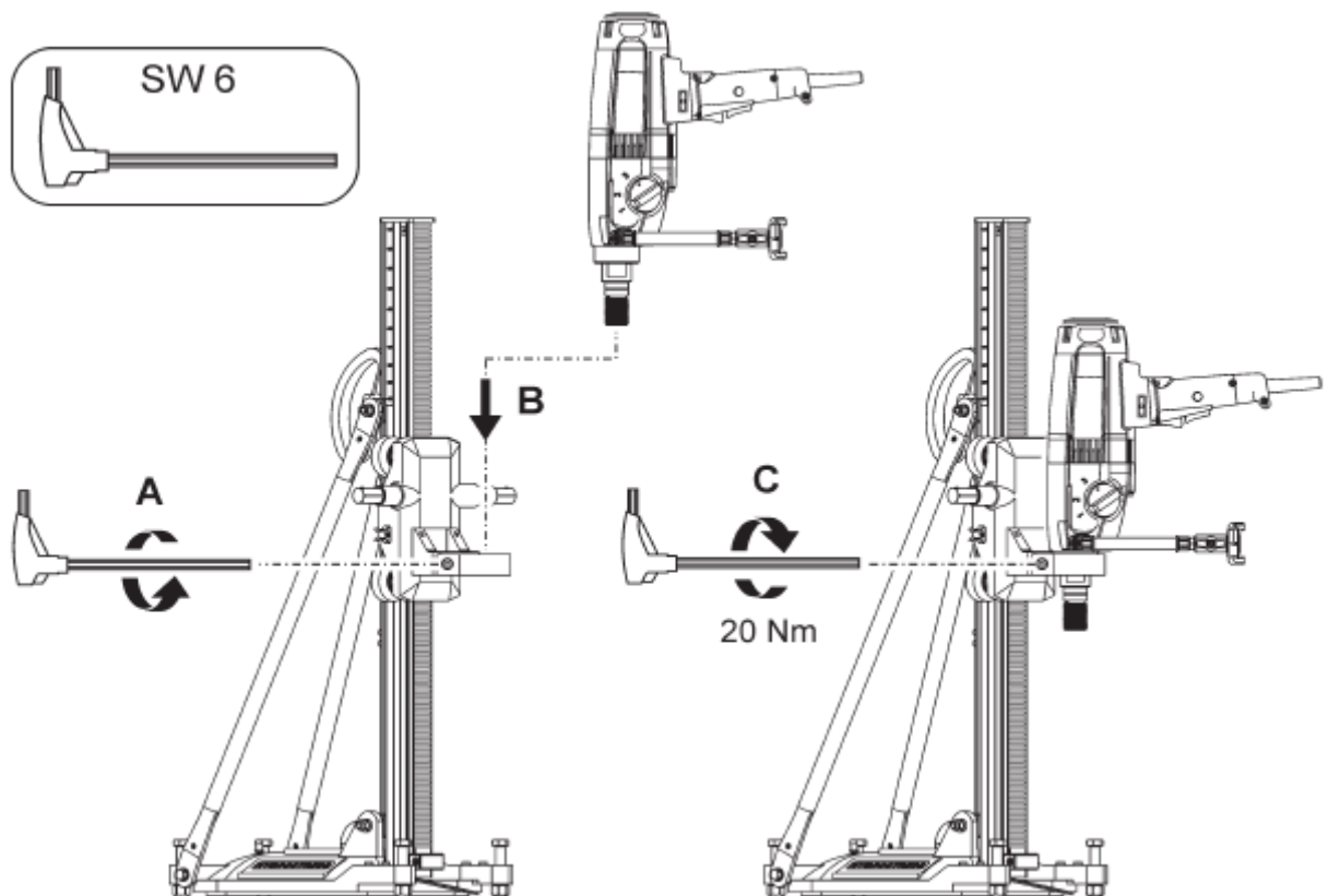
Подсоединение бурильной каретки
