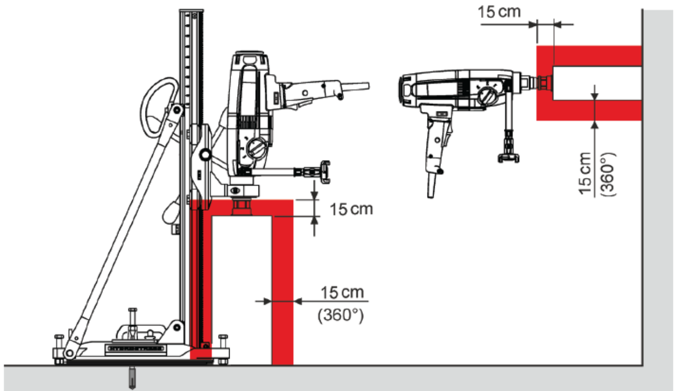
Зона опасности на электрическом оборудовании
